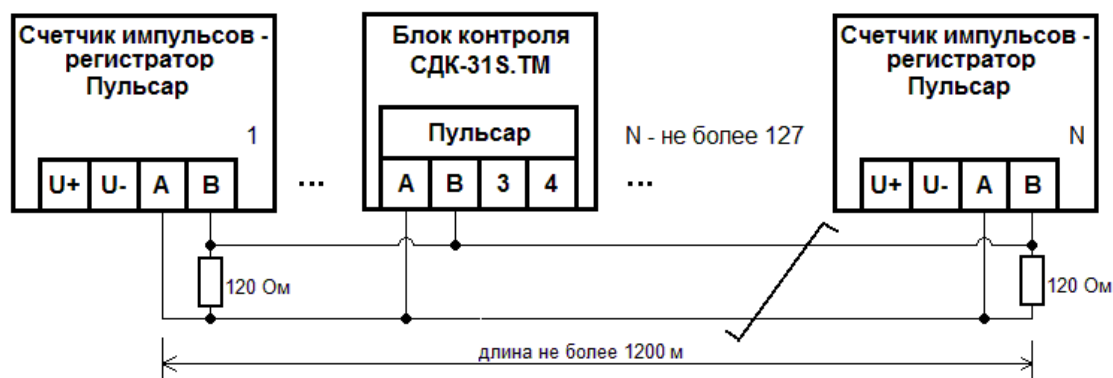
Рисунок 4. Подключение счетчиков импульсов – регистраторов «Пульсар», блок контроля СДК-31S.TM расположен в середине линии связи.
