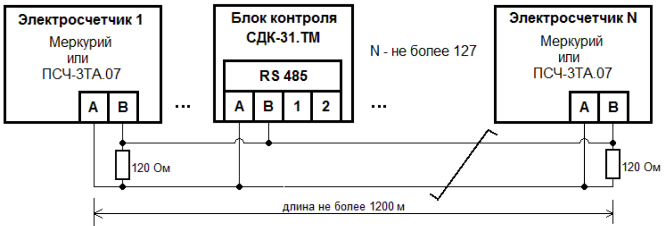
Рисунок 6. Подключение электросчетчиков, блок контроля СДК-31S.ТМ расположен в середине линии связи.
