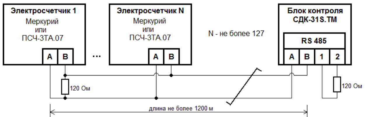
Рисунок 5. Подключение электросчетчиков, блок контроля СДК-31S.ТМ расположен на конце линии связи.
