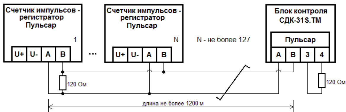
Рисунок 3. Подключение счетчиков импульсов – регистраторов «Пульсар», блок контроля СДК-31S.ТМ расположен на конце линии связи.
